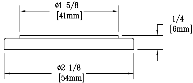
FLANGE
